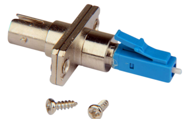
FOA-STF-LCM
